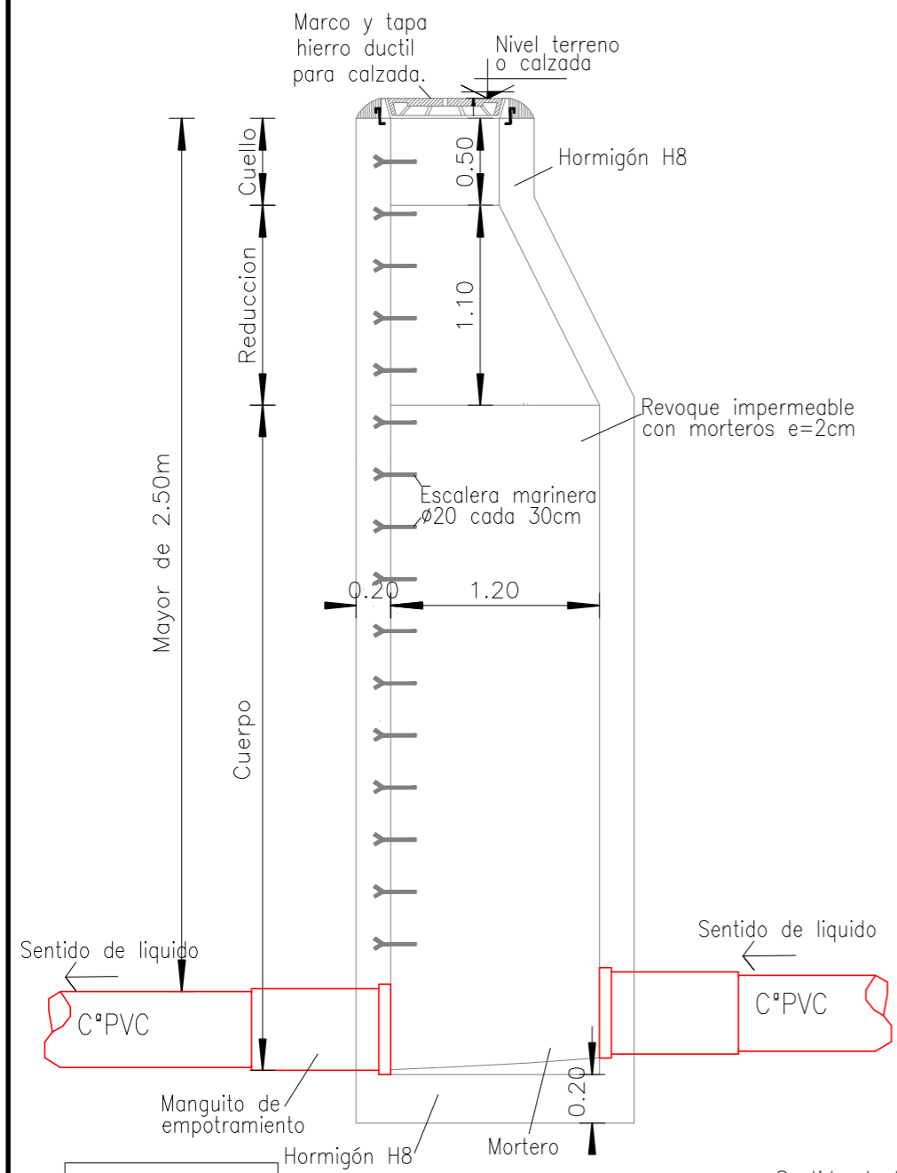
CORTE
