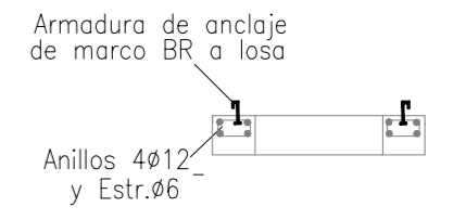
ARMADURA CABEZA DE BR.
