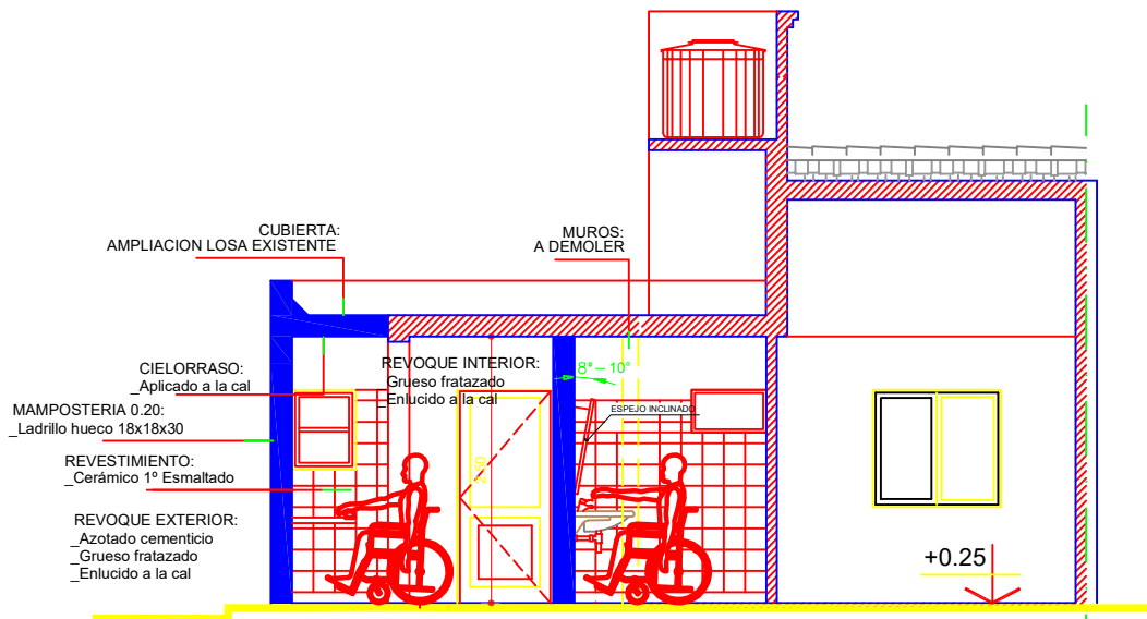
CORTE 2-2
