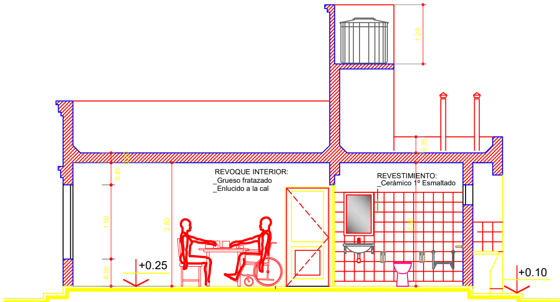
CORTE 1-1
